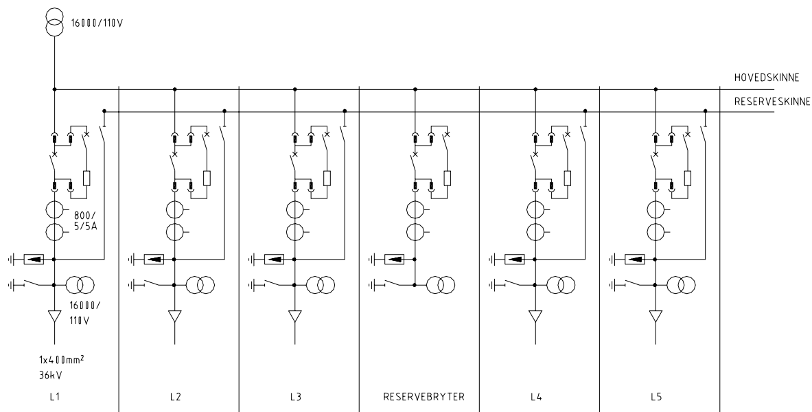
Figur 6.2 Typisk enlinjeskjema for koblingshus med prøvekrets for hver avgang.
