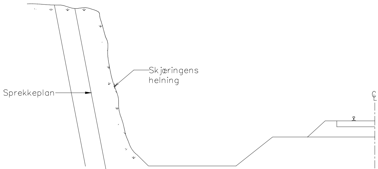
Figur 6.5 Tilpasning av skjæringshelning til sprekkplan
