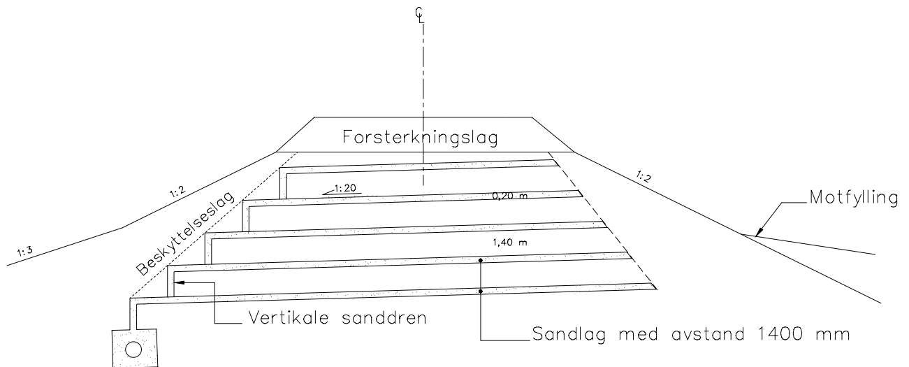
Figur 6.4 Prinsippskisse av leirfylling
