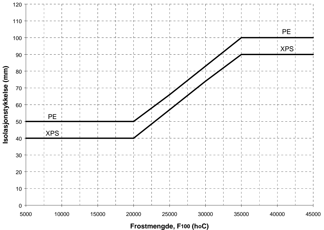
Figur 12.3 Krav til isolasjonstykkelse ved gitt frostmengde
