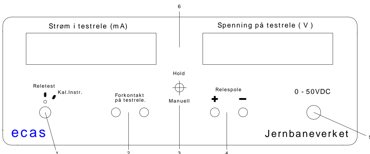
Figur 5.a.1 Frontplate på relétester
