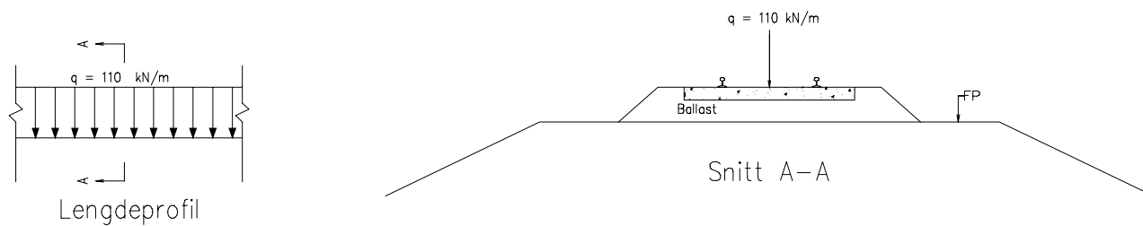
Figur 4.1 Dimensjonerende linjelast for enkeltsporet jernbane
