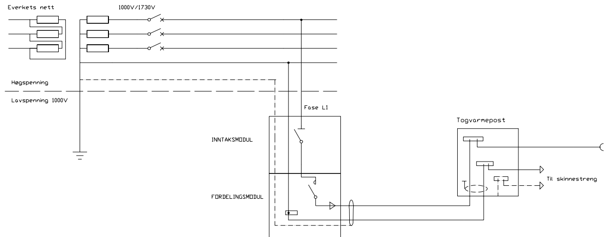
Figur 6.3 Eksempel på prinsipp for 50Hz togvarmeanlegg med 1000V/1730V transformator, 1000V inntaksmodu, en fordelingsmodul og en togvarmepost.
