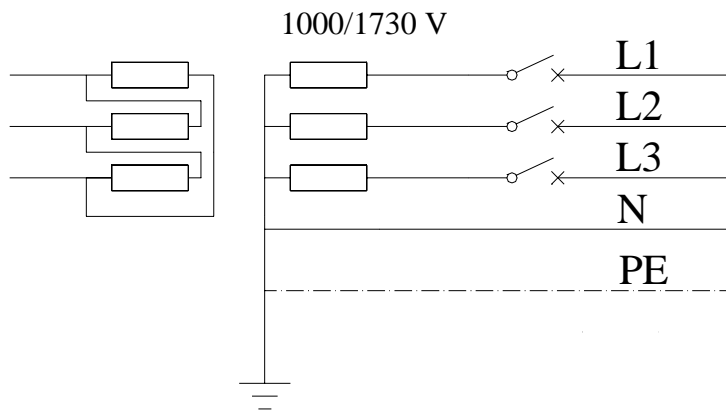
Figur 6.1 Kobling av togvarmetransformator med direkte jordet nullpunkt, 1000 / 1730 V.
