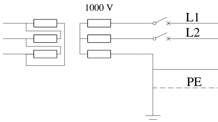
Figur 6.2 Kobling av togvarmetransformator med direkte jordet ene fasen, 1000 V.
