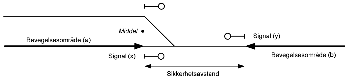
Figur 6.13 Motrettede bevegelsesområder
