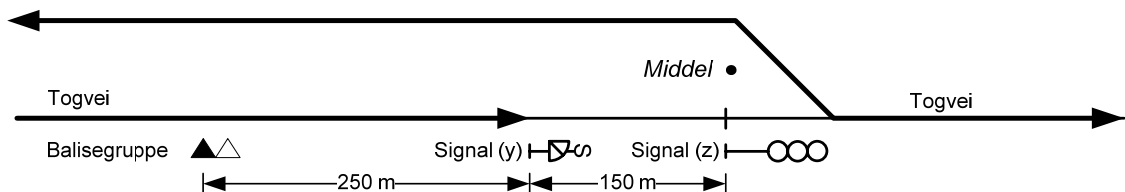
Figur 6.11 Samtidige togveier med sikkerhetsavstand 150 meter
