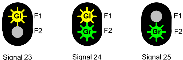
Figur 6.18 Forsignal - signalbilder
