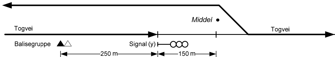
Figur 6.10 Samtidige togveier med sikkerhetsavstand 150 meter
