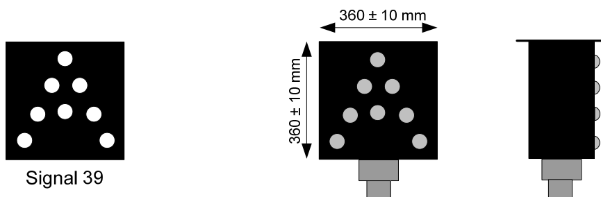
Figur 6.30 Kjøretillatelse "A-signal" - signalbilde og eksempel på lyssignal
