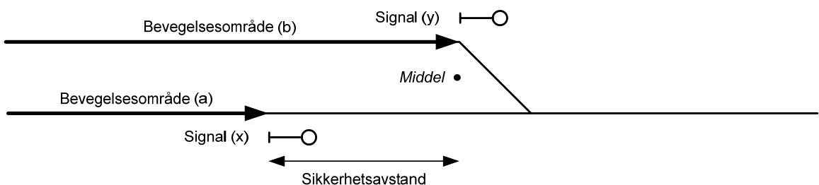
Figur 6.12 Parallele bevegelsesområder
