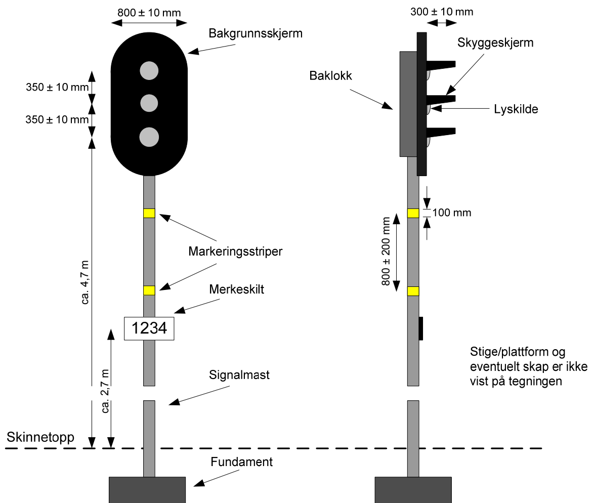
Figur 6.17 Eksempel på 3-lys hovedsignal
