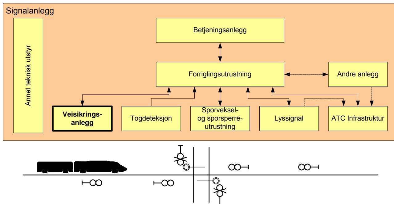
Figur 9.1 Systemoversikt signalanlegg
