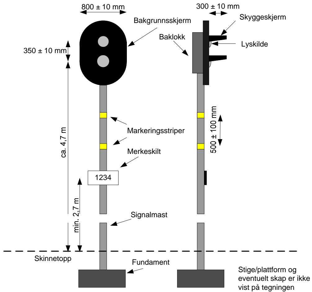
Figur 12.7 Enkeltinnkjørsignal
