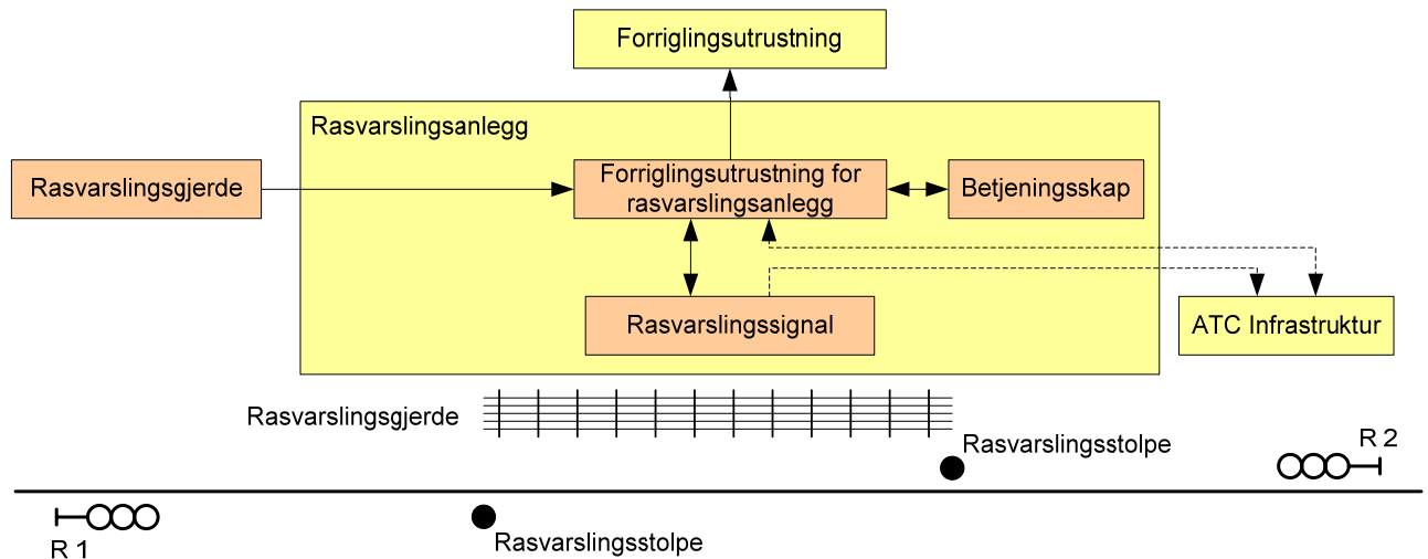
Figur 12.2 Systemdefinisjon rasvarslingsanlegg
