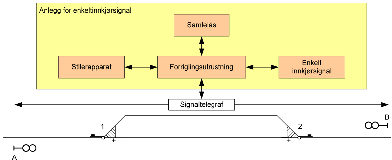
Figur 12.5 Systemdefinisjon anlegg for enkelt innkjørsignal
