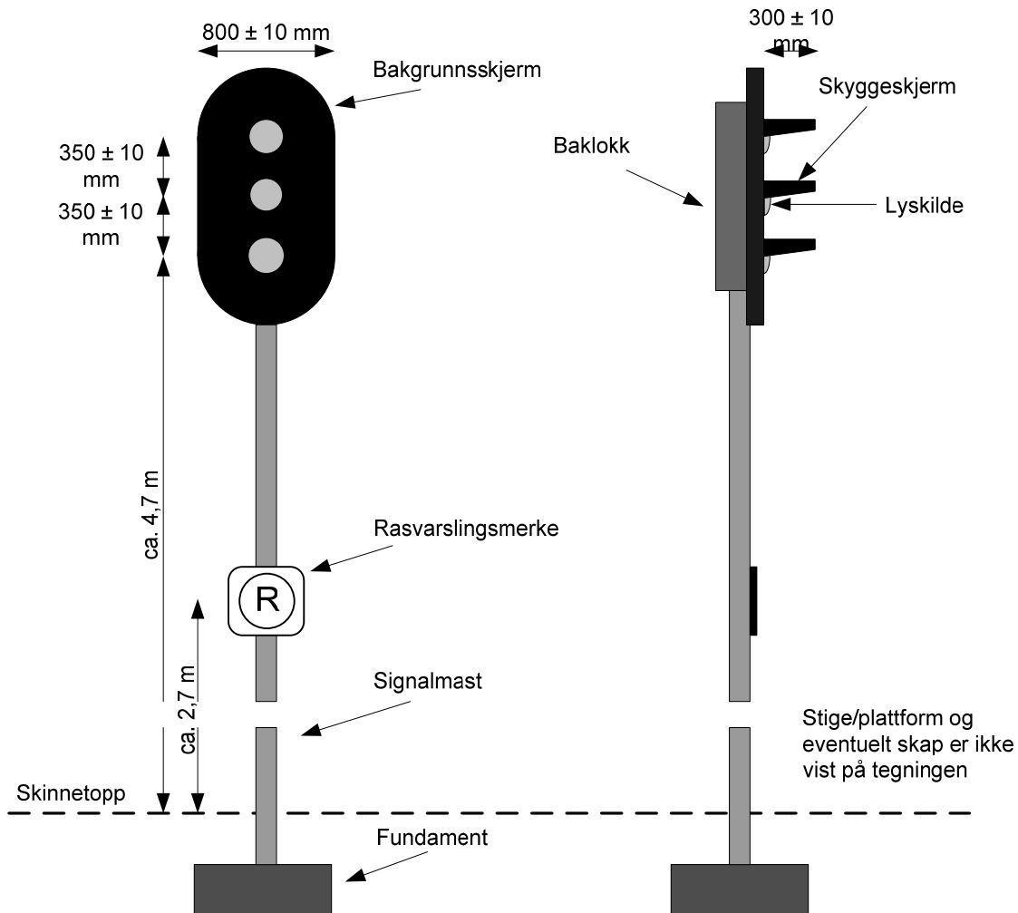
Figur 12.4 Rasvarslingssignal
