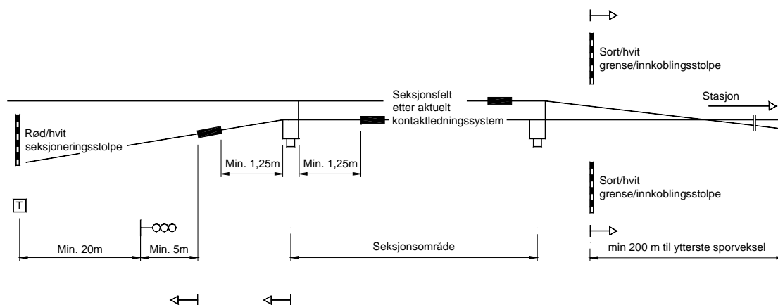
Figur 6.6 Prinsippsskisse for plassering av seksjonsfelt i forhold til hovedsignal, enkeltsporet strekning, seksjonsfelt over 3, 4 og 5 spennlengder.
