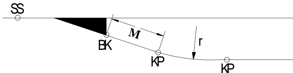
Figur 5.5 Krav til rettlinje M ved linjedelende veksel
