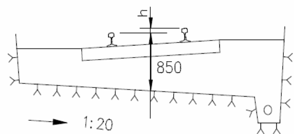
Overgangskurver og sirkelkurver med overhøyde
