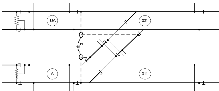
Figur 7.a.7 Overkjøringsspor uten eget sporavsnitt - enkeltisolert sporfelt - Hovedspor elektrisk adskilt
