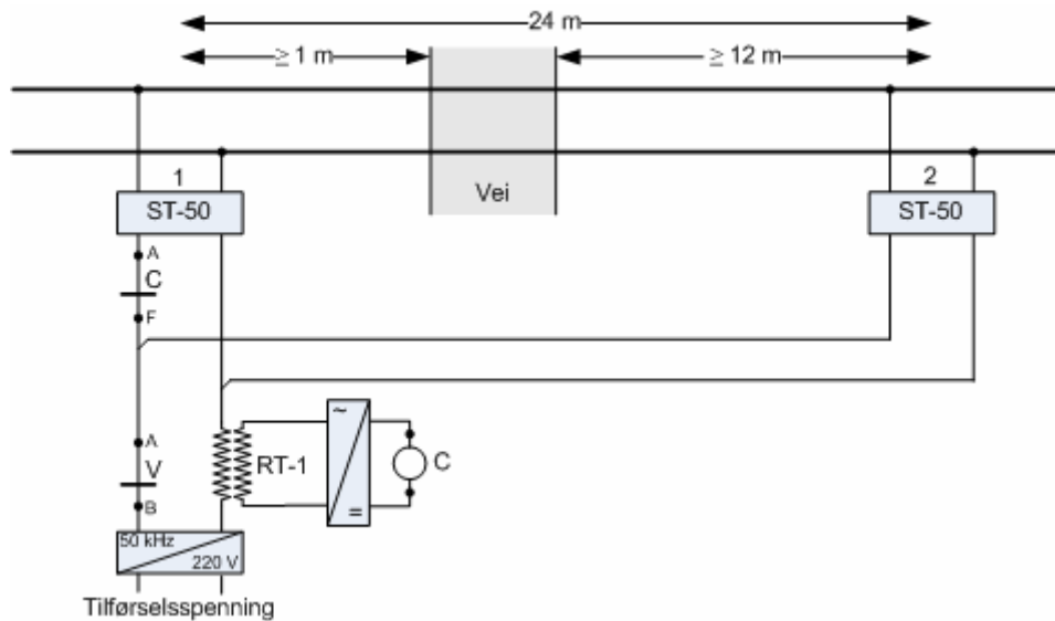
Figur 7.c.4 50 kHz Utløsningsfelt
