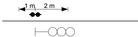
Figur 7.f.8 Hovedsignal eller dvergsignal ved isolert skjøt
