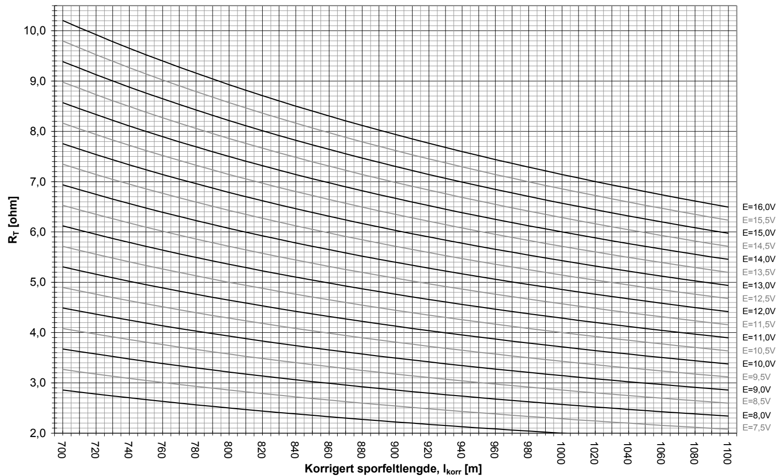
Figur 7.b.9 Diagram for å bestemme forholdet mellom tilførselsspenning/-motstand for likestrømsporfelter, Type 2 og 3.
