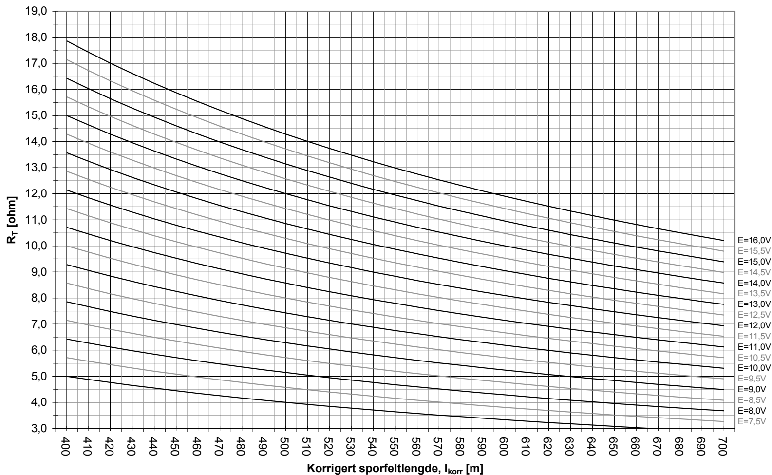
Figur 7.b.8 Diagram for å bestemme forholdet mellom tilførselspenning/-motstand for likestrømsporfelter, Type 2 og 3.
