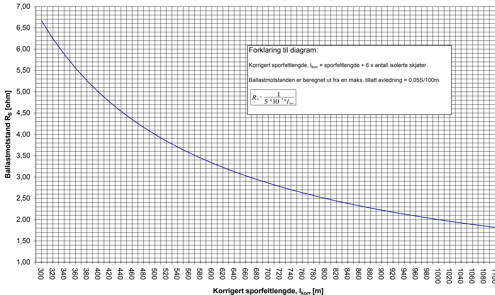
Figur 7.b.6 Forhold mellom sporfeltlengde, antall isolerte skjøter og ballastmotstand for likestrømsporfelter, Type 1 og 2 (Lengde > 300 meter)
