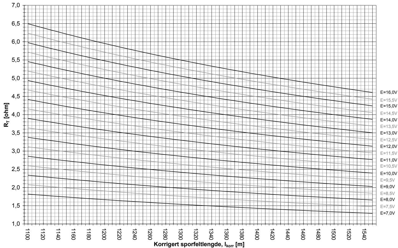
Figur 7.b.10 Diagram for å bestemme forholdet mellom tilførselsspenning/-motstand for likestrømsporfelter, Type 3.
