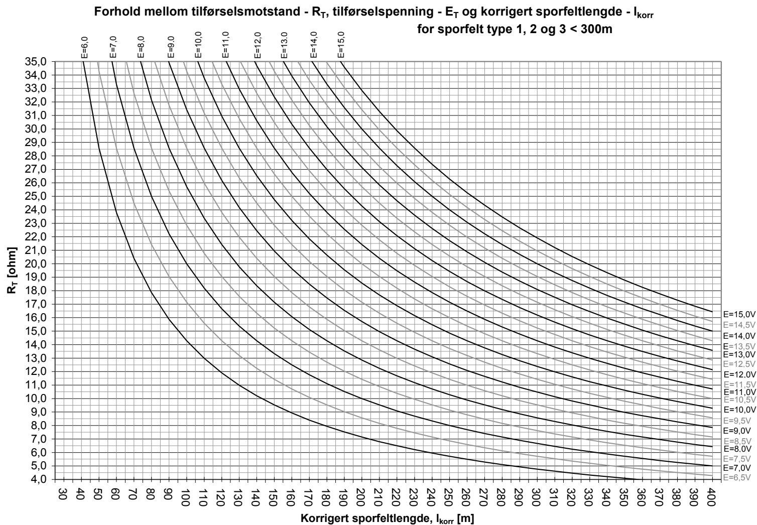
Figur 7.b.7 Diagram for å bestemme forholdet mellom tilførselsspenning/-motstand for likestrømsporfelter, Type 1, 2 og 3.
