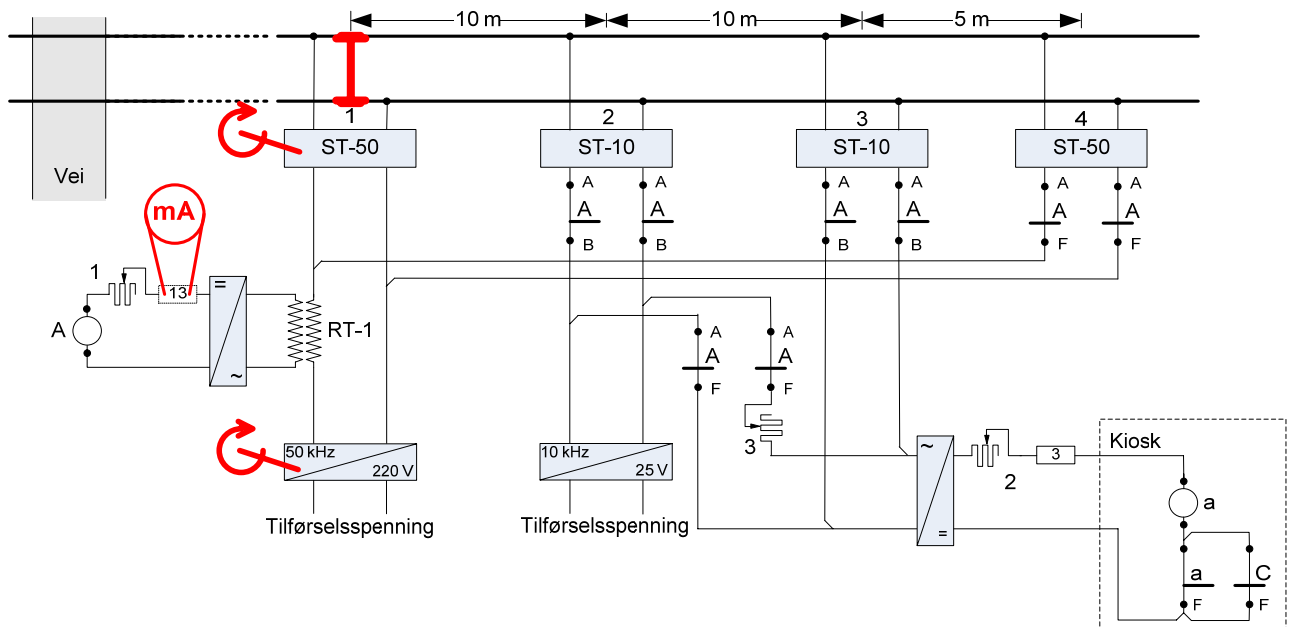
Figur 7.c.1 Innkoblingsfelt - justering av 50 kHz tilførsel og skilletransformator 1
