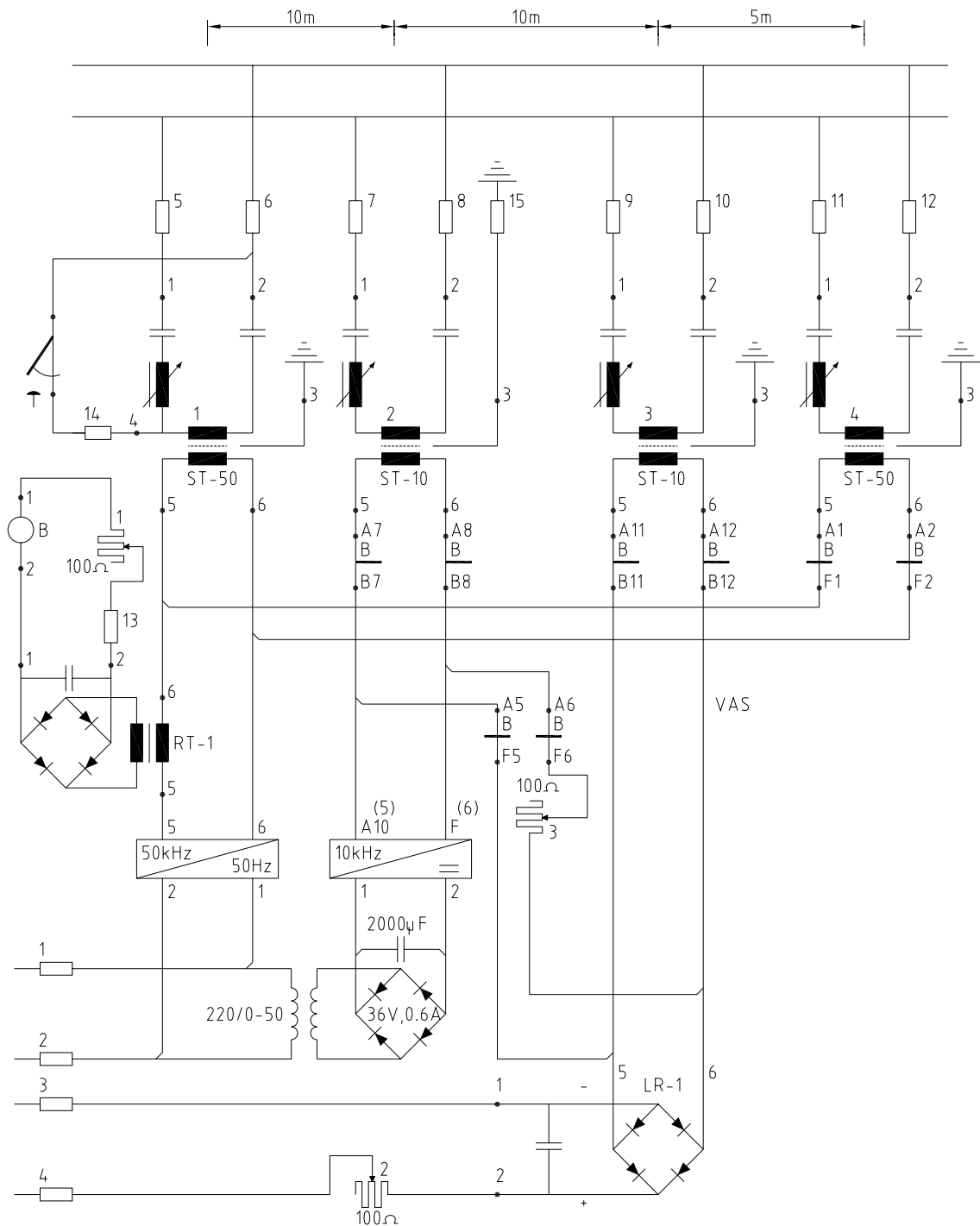
Figur 7.c.10 Veiledende kretsskjema for 10/50 kHz innkoblingsfelter, relé type JRS
