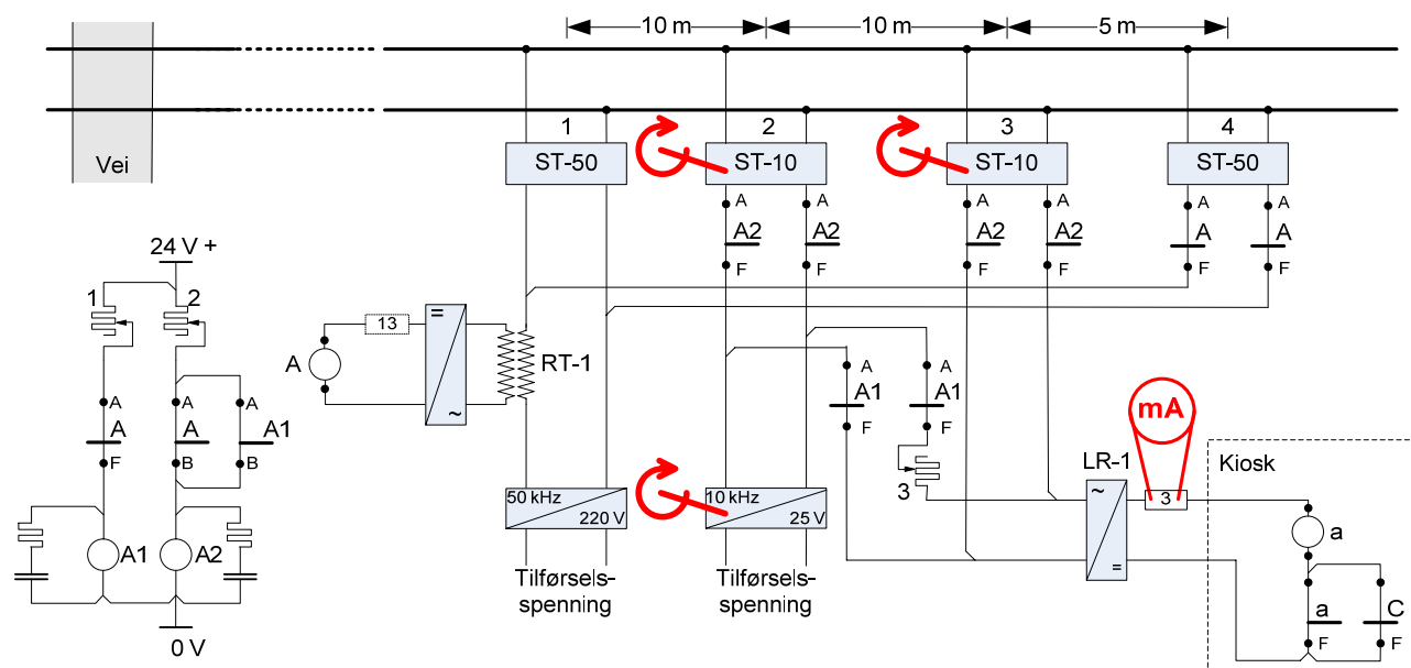
Figur 7.d.5 Innkoblingsfelt - justering av 10 kHz
