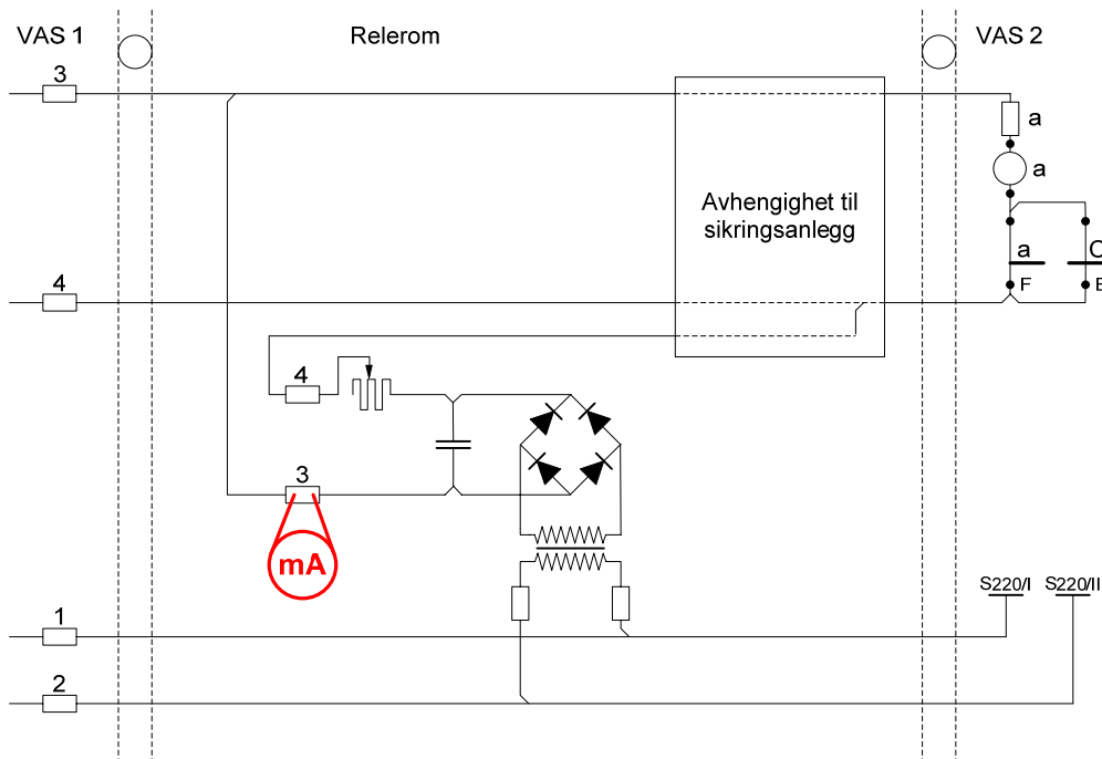
Figur 7.d.9 Tilleggsstrømforsyning
