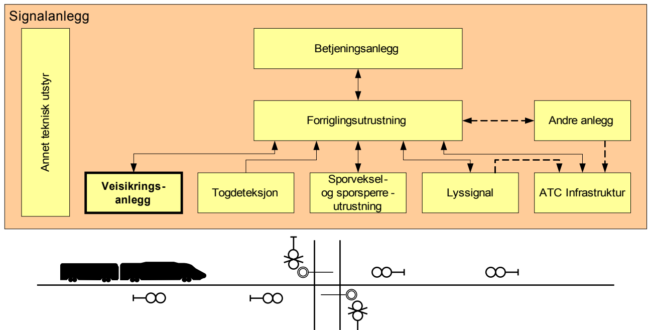
Figur 9.1 Systemoversikt signalanlegg
