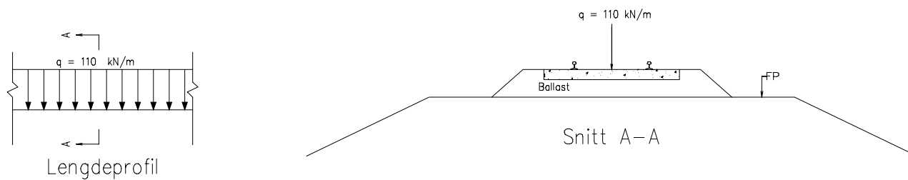
Figur 4.1 Karakteristisk linjelast for enkeltsporet jernbane
