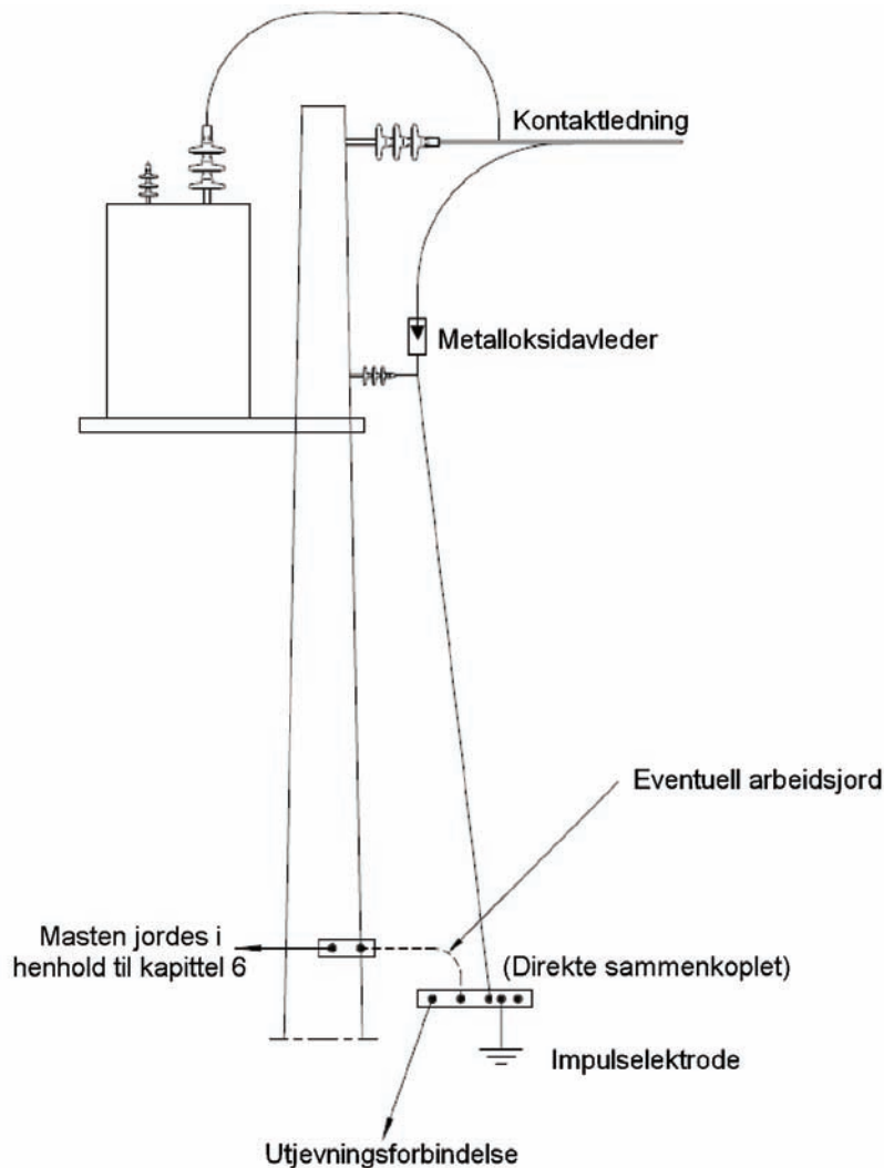
Figur 7.1 Overspenningsvern ved sugetransformator, reservestrømstransformator og kabelendemuffe
