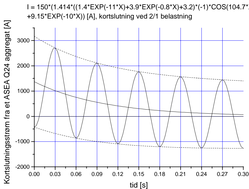
Figur 11 Kortslutningsstrøm fra et Q24 aggregat i fullast
