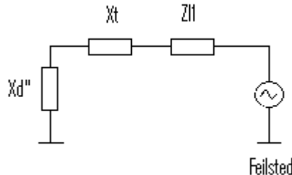
Figur 21 Kortslutningskrets for den roterende omformeren
