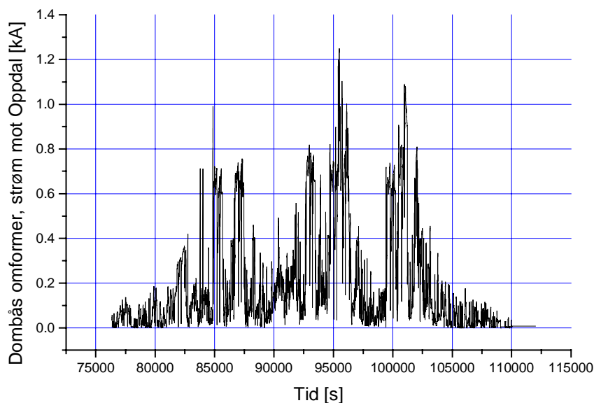
Figur 23 Belastningsstrøm utgående linje på Dombås mot Oppdal
