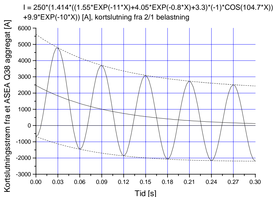
Figur 13 Kortslutningsforløp fra et Q38 aggregat ved kortslutning fra fullast
