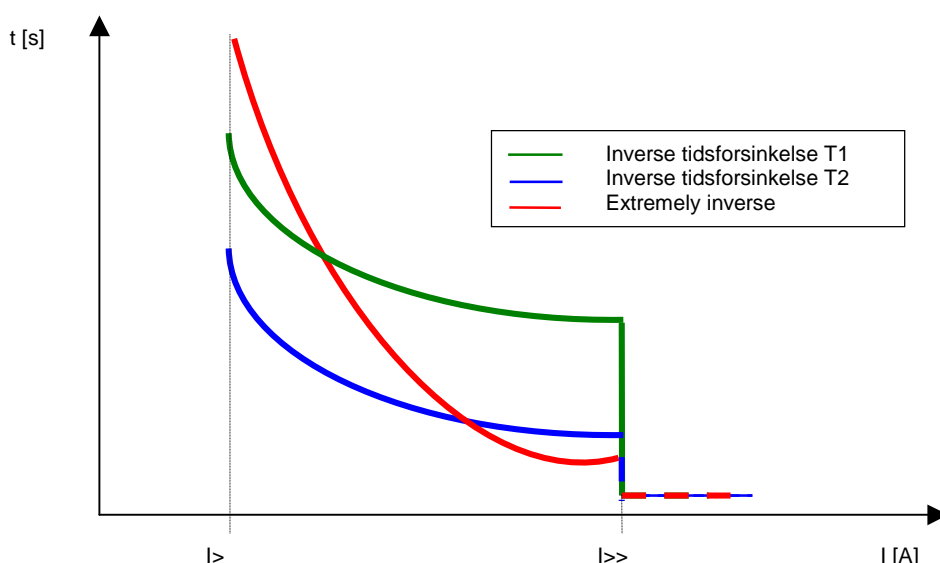
Figur 7 Invers og extremely invers karakteristikk
