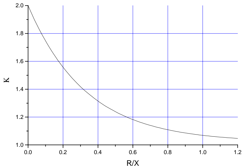
Figur 9 Faktor \kappa for seriekretser som en funksjon av forholdet mellom R og X
