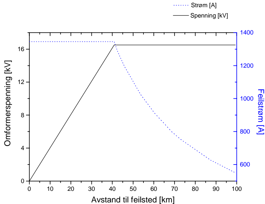
Figur 17 Feilstrøm og spenning fra et statisk omformeraggregat
