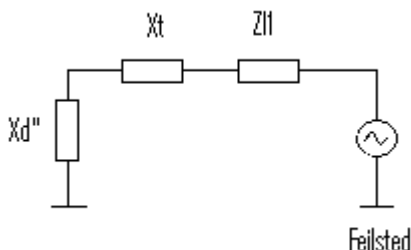
Figur 21 Kortslutningskrets for den roterende omformereren
