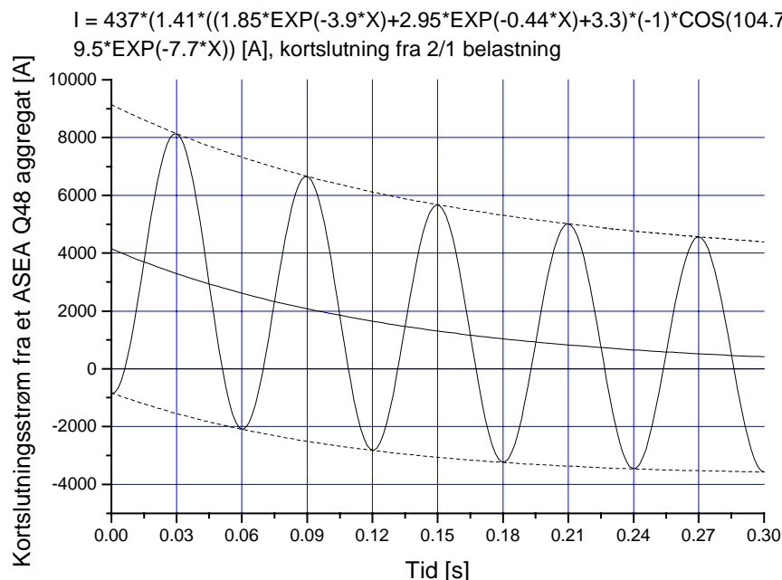
Figur 15 Kortslutningsforløp fra et Q48 aggregat ved kortslutning fra fullast
