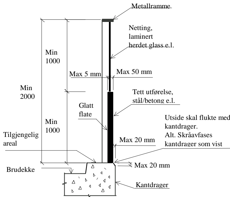
Figur 10.1 Generelle krav til beskyttelsesskjerm. Snitt
