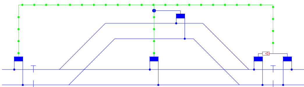
Returledning over stasjoner med dobbeltisolerte sporfelter
