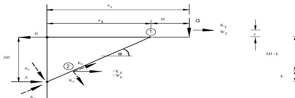
Figur 15.1 Krefter og belastninger på utligger
