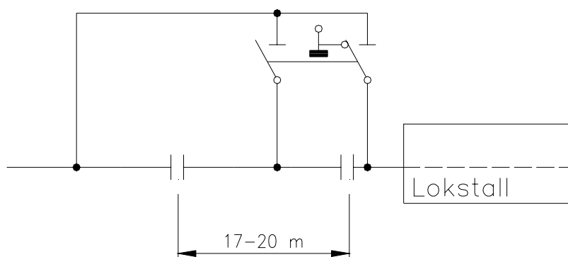
Figur 6.3 Beskyttelsesseksjon foran lokomotivstall og lignende.
