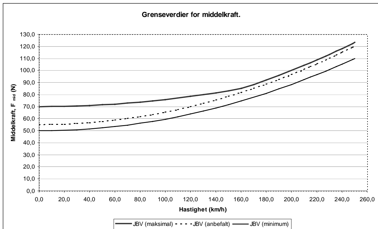
Figur 5.d.1 Middelkraft som funksjon av togfremføringshastighet.
