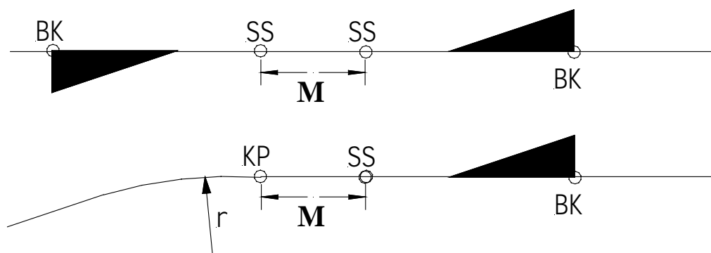
Figur 5.4 Krav til rettlinje M mellom to motstående veksler/veksel og curve
