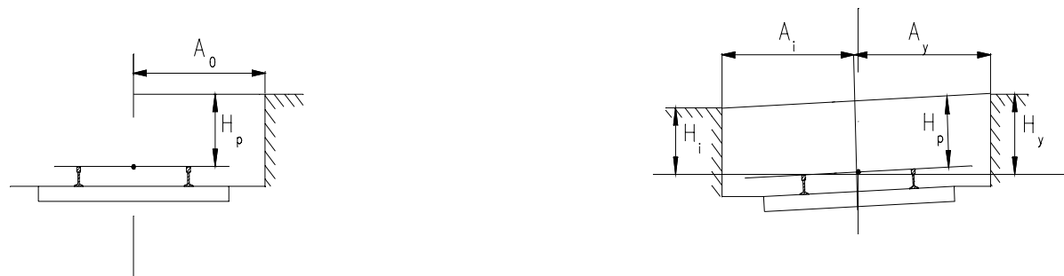
Figur 14.1 Plattformhøyder og avstand spormidt - plattformkant
