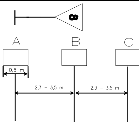
Figur 10.13 Baliseplassering ved hastighetssignaler.
