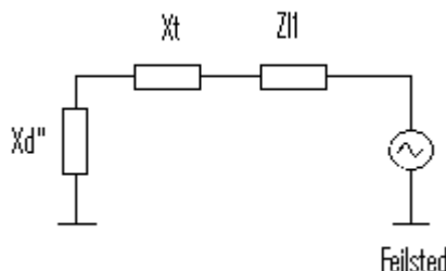
Figur 21 Kortslutningskrets for den roterende omformeren
