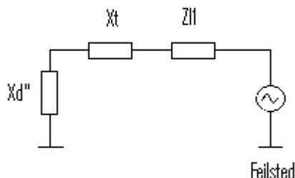
Figur 21 Kortslutningskrets for den roterende omformereren
