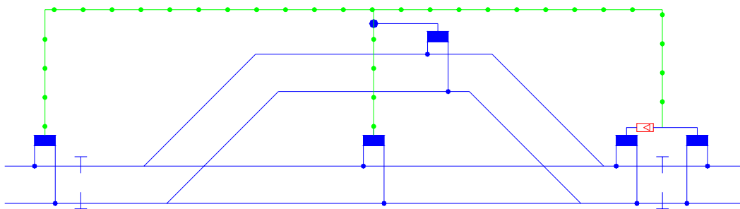
Returledning over stasjoner med dobbeltisolerte sporfelter
