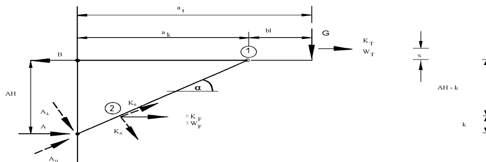
Figur 15.1 Krefter og belastninger på utligger
