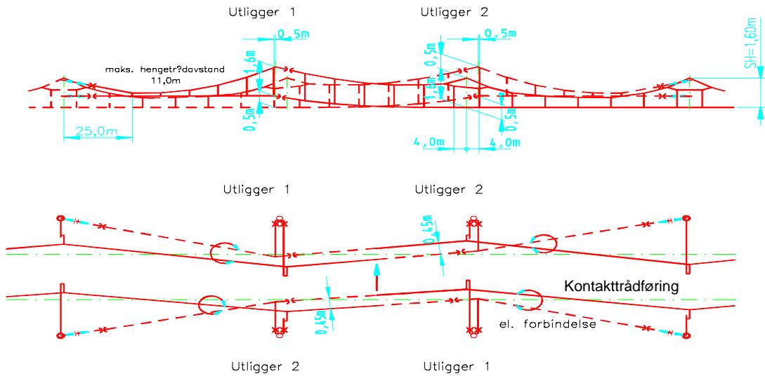
Figur 5.c.11 3-felts seksjon
