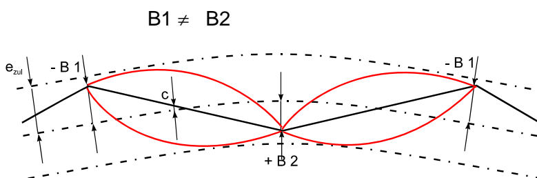
Figur 5.c.14 Kontakttrådens sikksakk i store kurver
