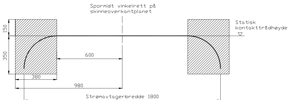
Figur 5.c.24 Klemmefritt rom.
