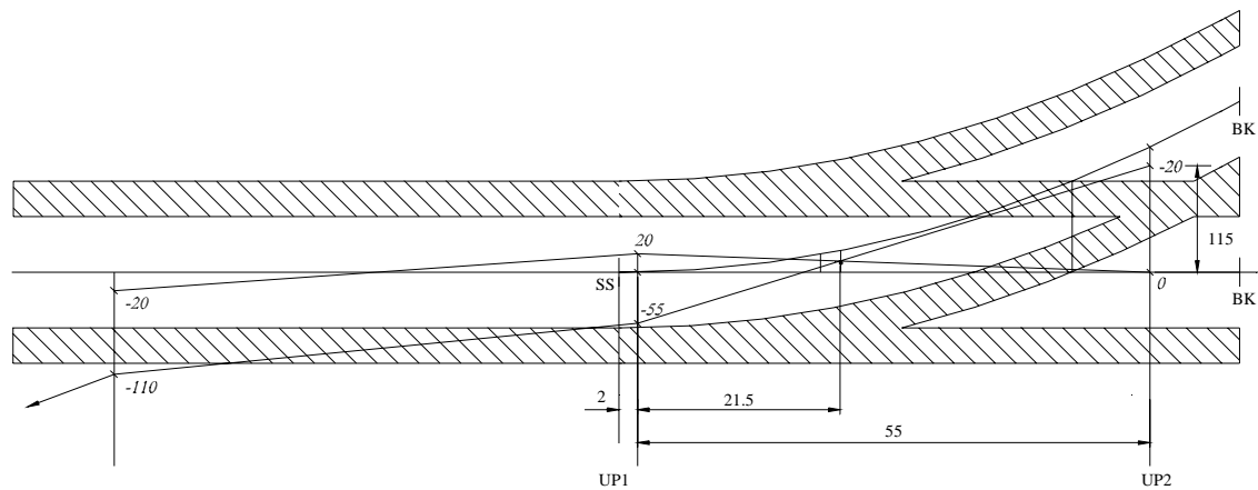
Figur 5.c.34 Ferdig prosjektert sporveksel for S20.
