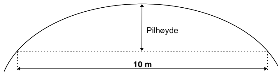
Figur 13.3 Definisjon av pilhøyde
