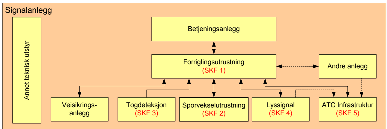
Figur 4.3 Sikkerhetskritiske funksjoner
