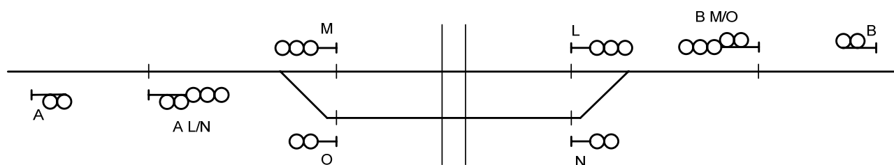
Figur 9.8 Planovergang mellom inn- og utkjørhovedsignalene.
