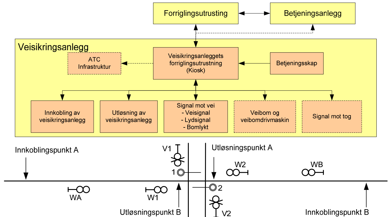
Figur 9.2 Systemdefinisjon veisikringsanlegg
