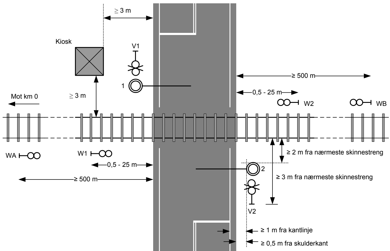
Figur 9.3 Plassering av utstyr for veisikringsanlegg
