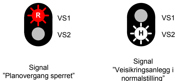
Figur 9.11 Veisignal - Signalbilder
