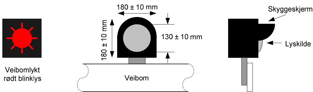
Figur 9.13 Veibomlykt
