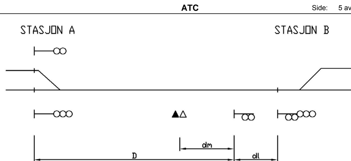
Figur 10.1 Plassering av lenkingsbalisegrupper på linjen
