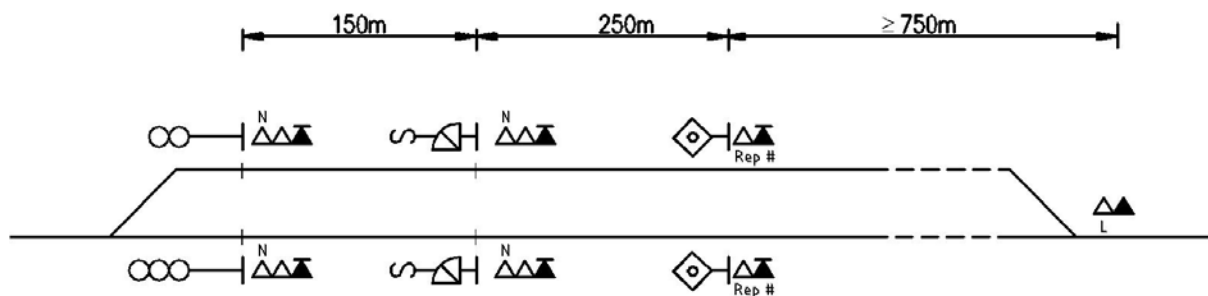
Figur 10.3 Samtidig innkjør - alternativ 2.
