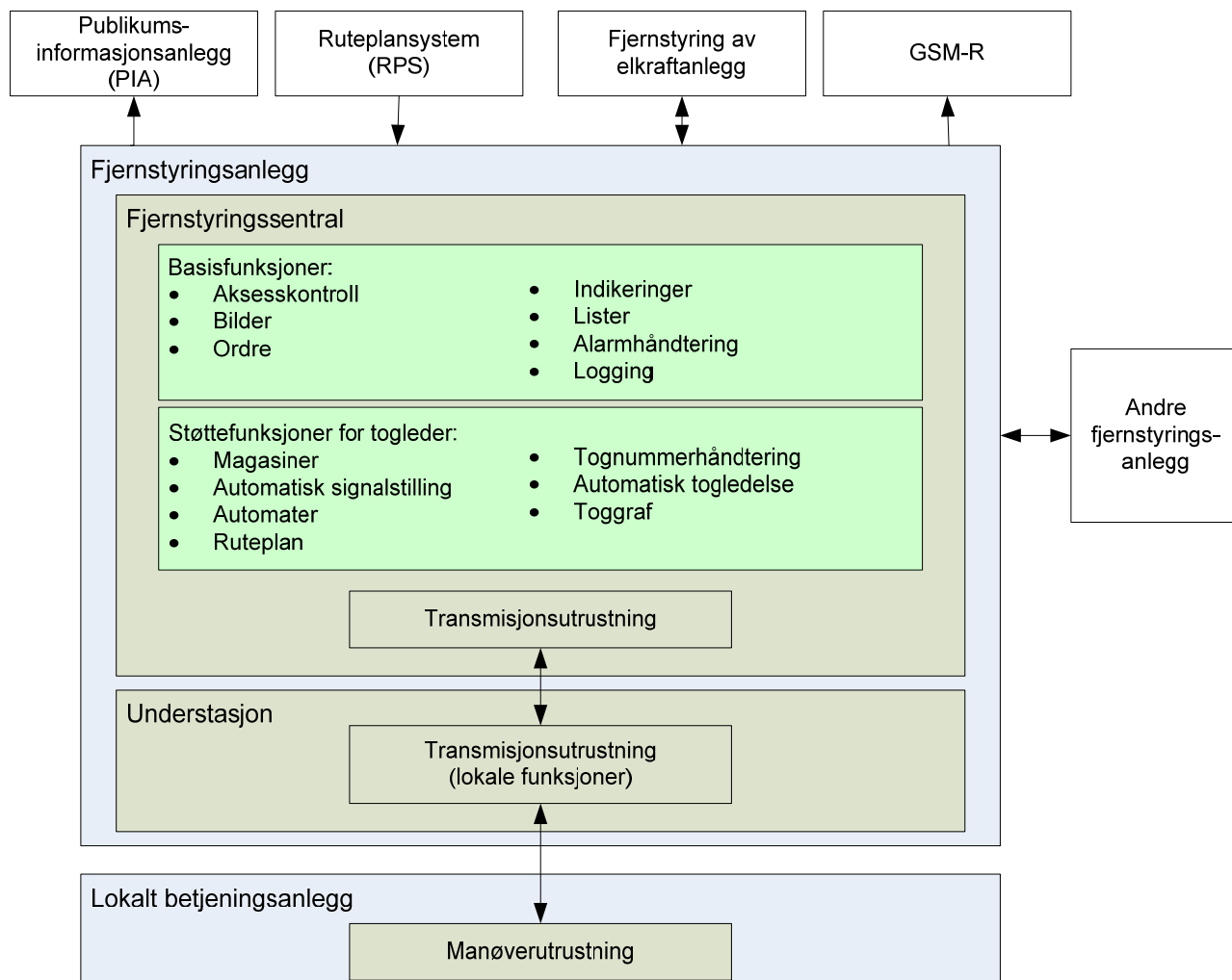
Figur 11.3 Systemdefinisjon fjernstyringsanlegg
