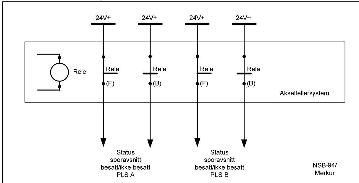
Figur 7.f.20 Grensesnitt mellom akselteller og sikringsanlegg NSB-94 og Merkur
