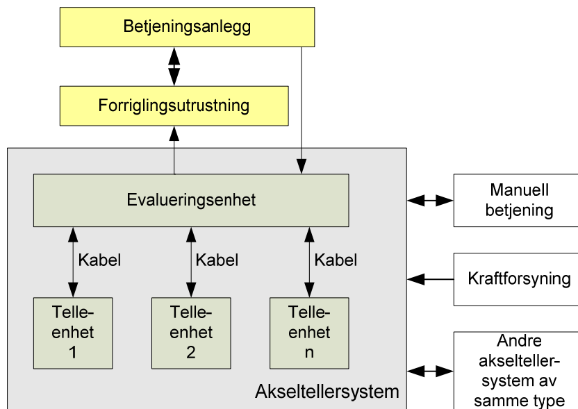
Figur 7.f.1 Systemoversikt akselteller
