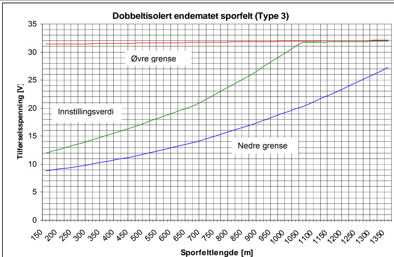
Figur 7.a.6 Dobbeltisolert endematet sporfelter, Type 3
