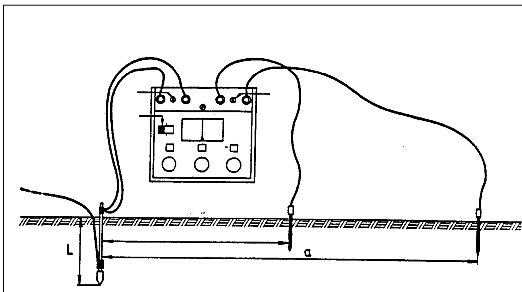
Figur 9.b.3 Skisse av for oppkopling av måleutstyr
