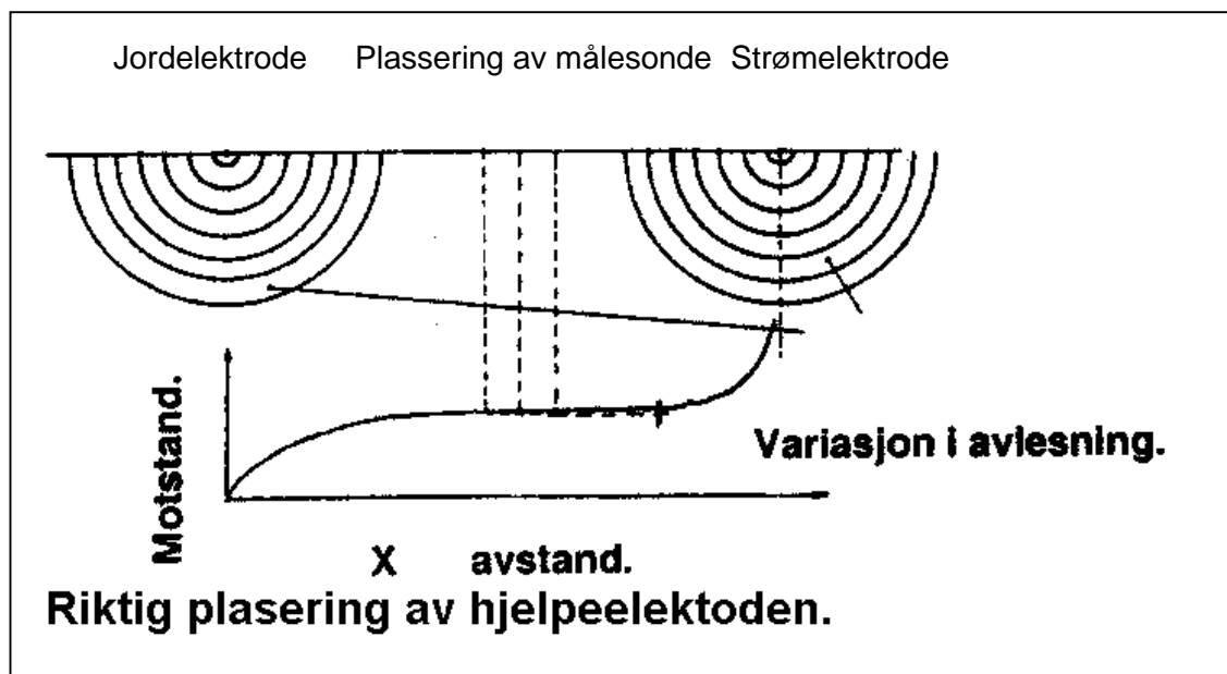
Figur 9.b.1 Måleoppsett
