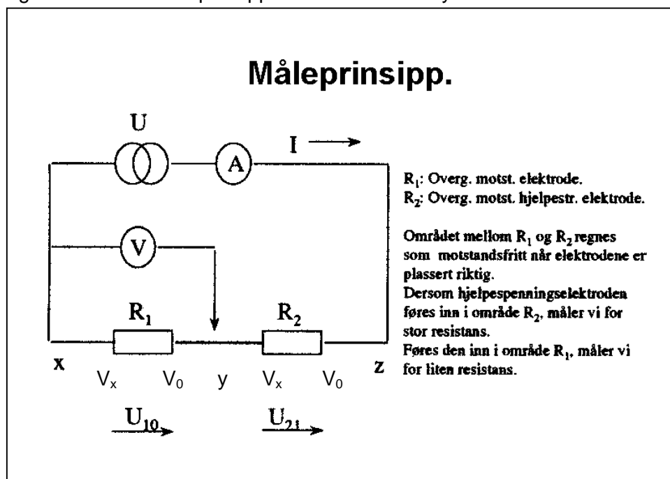
Figur 9.b.2 Måleprinsipp med elektriske symboler
