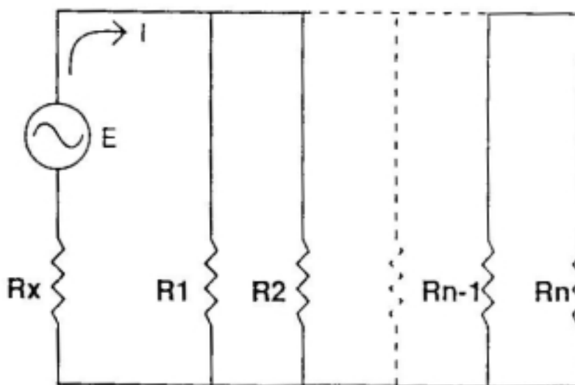
Figur 9.b.4 Prinsipp for måling av jordovergangsmotstand ved hjelp av jordsystemmåler
