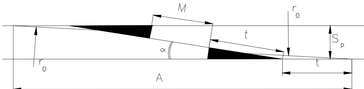
Figur 5.5 Sporsløyfe
