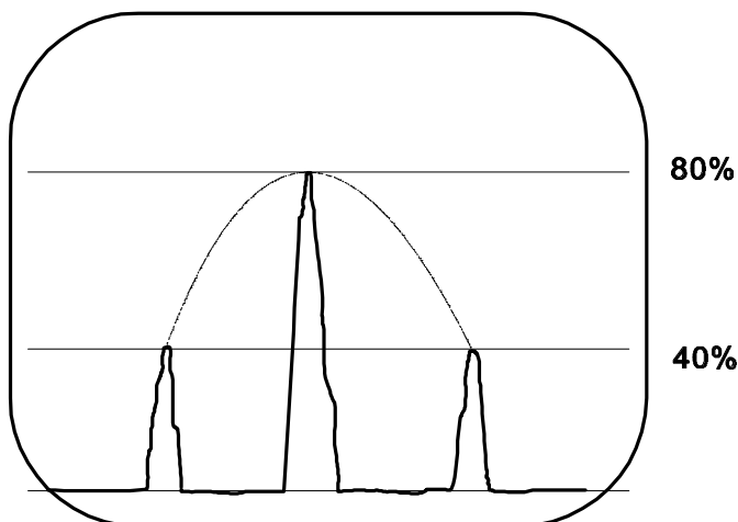
Figur 7.b.1 Beregning av feilutbredelse ved tandemmetoden
