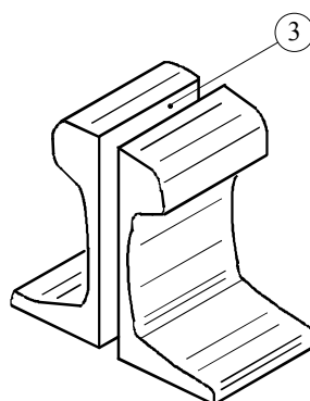
Figur 11g.2 Uttak av prøveemner - lengdesnitt
