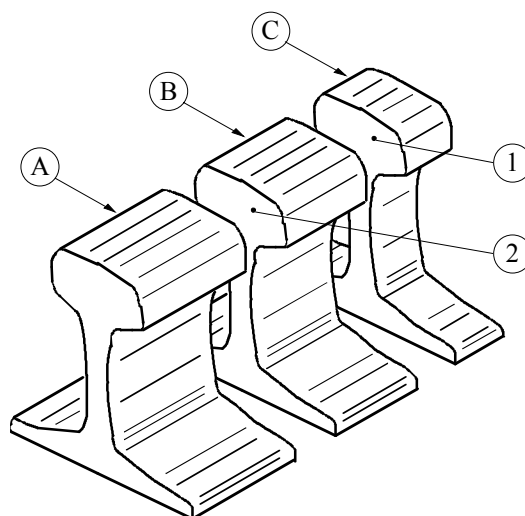
Figur 11g.1 Uttak av prøveemner - tverrsnitt
