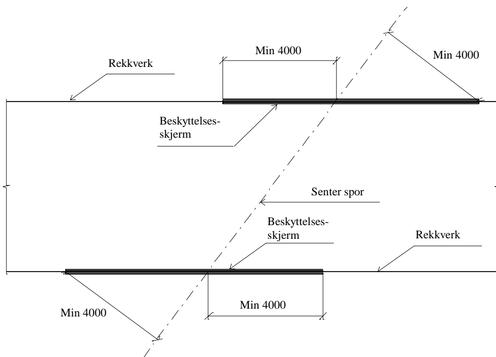
Figur 10.2 Krav til utstrekning av beskyttelsesskjerm. Plan
