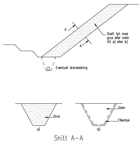
Figur 11.5 Skråningsgrøfter vinkelrett på linjeretningen
