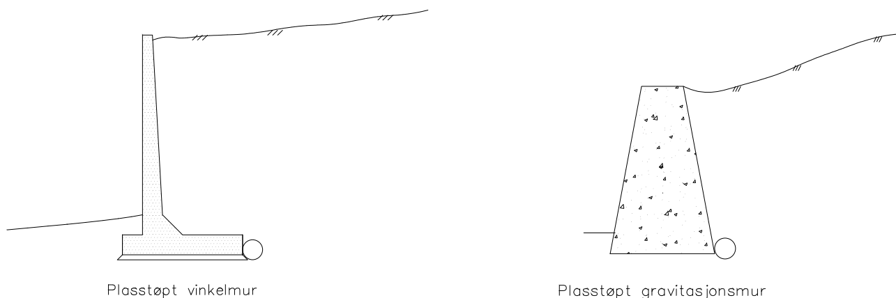
Figur 6.4 Plasstøpt vinkelmur og plasstøpt gravitasjonsmur
